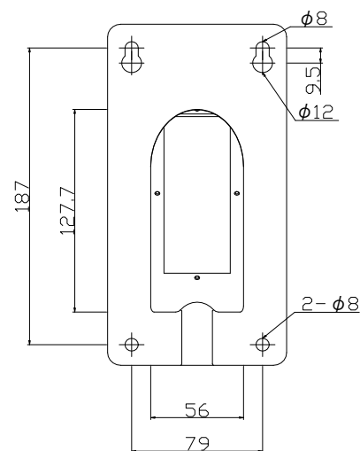
【壁付けブラケット壁面寸法】
