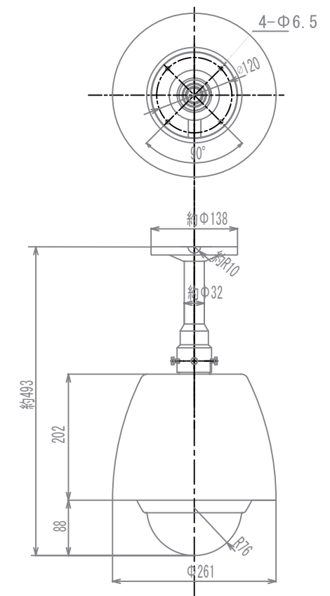
AT-R950POE/R950DC 外観図
